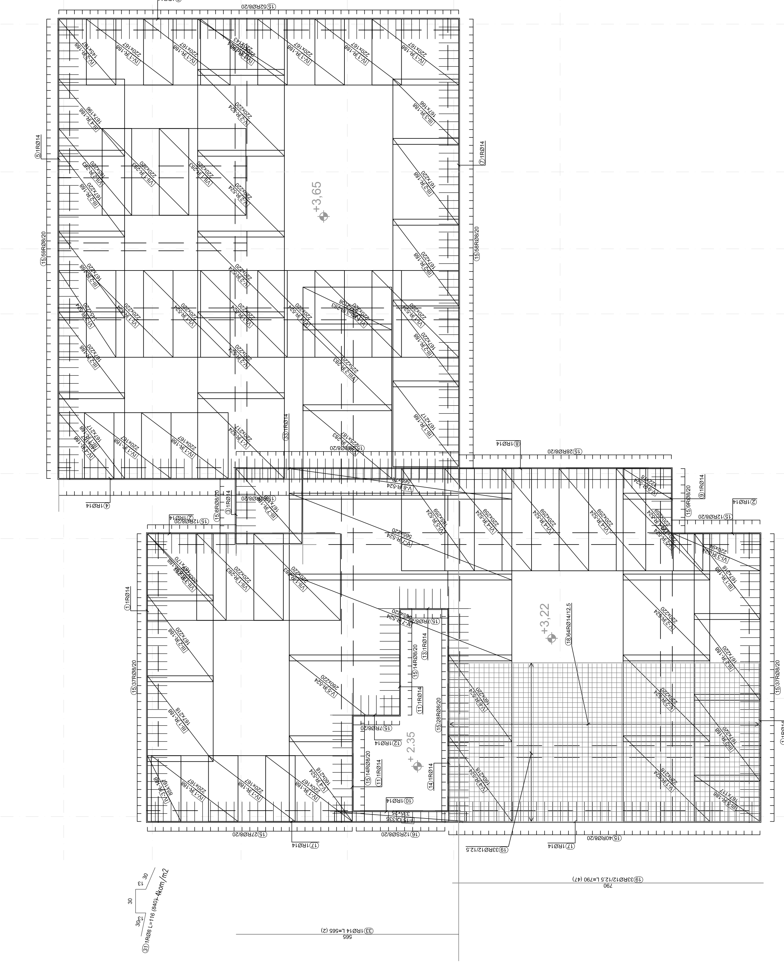
AB PLOŠČA POZ 10; d=20cm zgornja armatura
