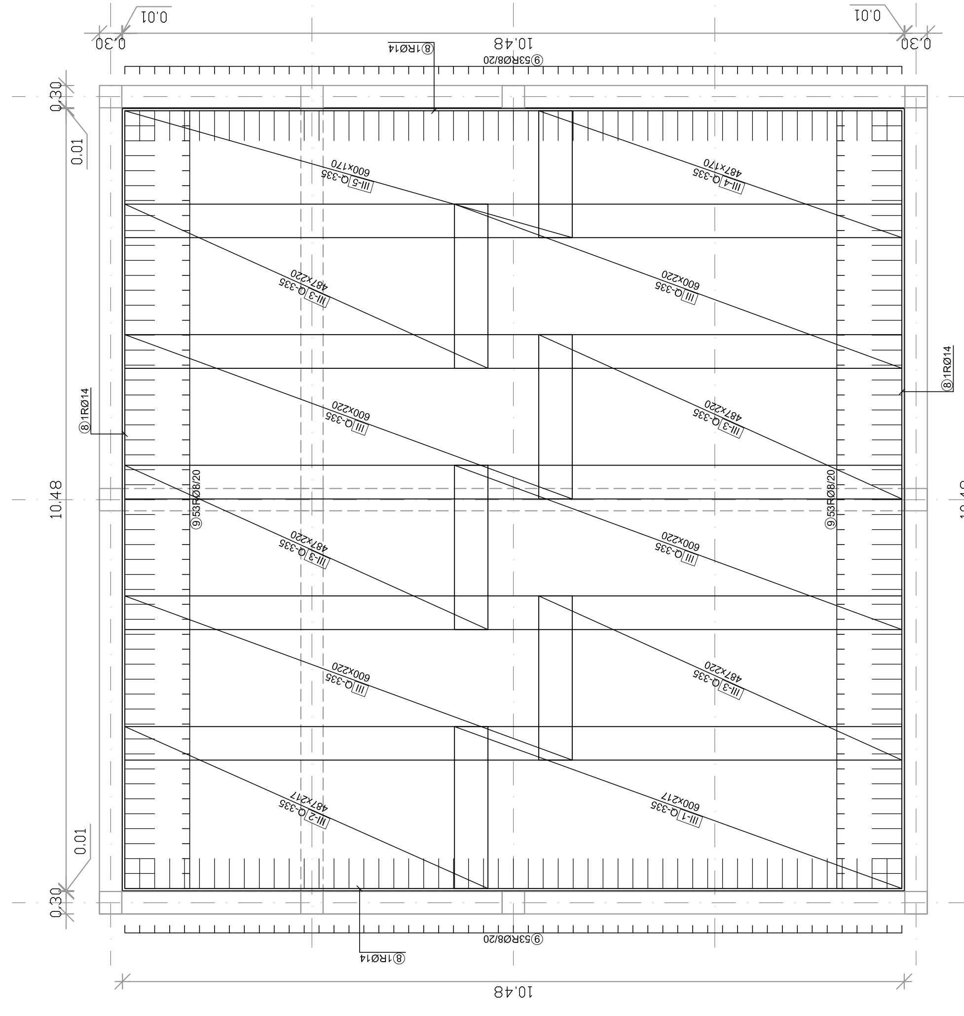
TALNA PLOŠČA; d=15cm – spodnja armatura
