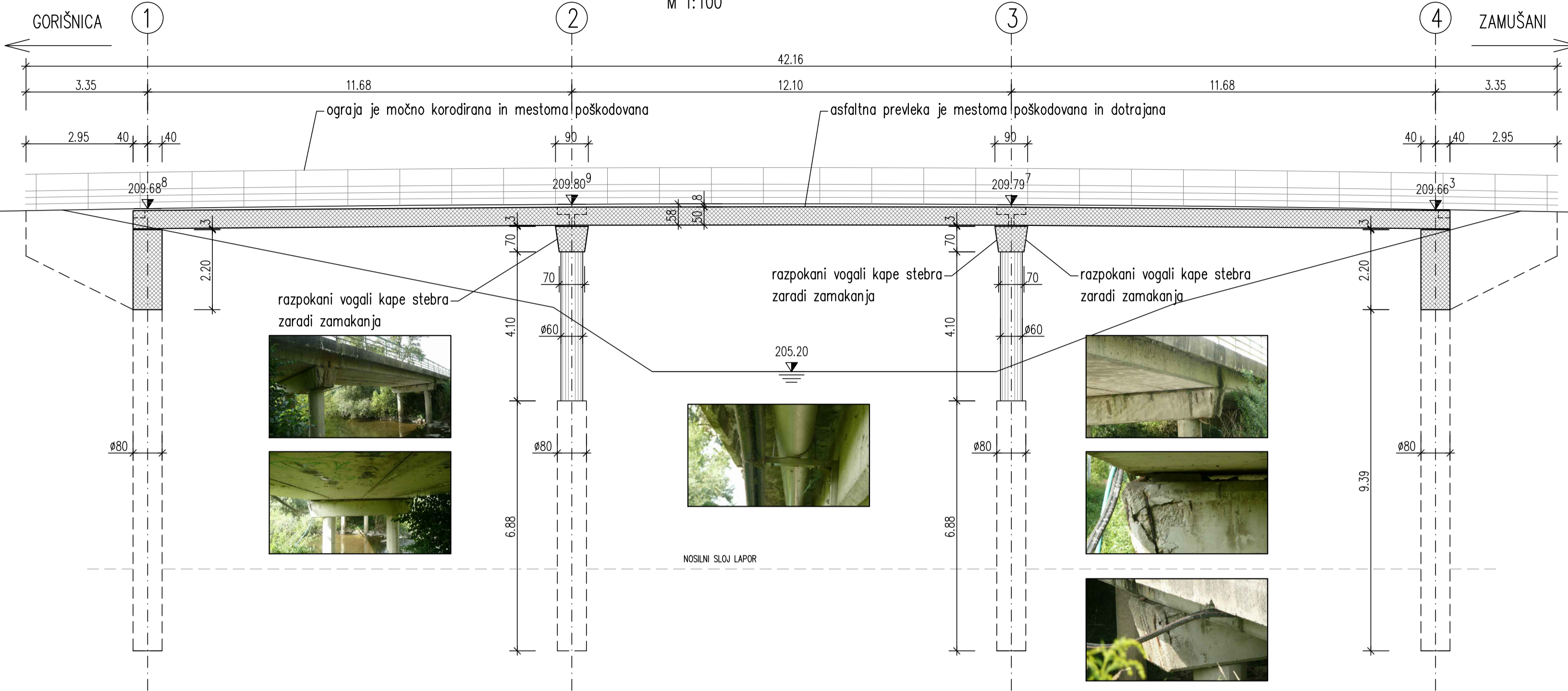
VZDOLŽNI PREREZ M 1:100
